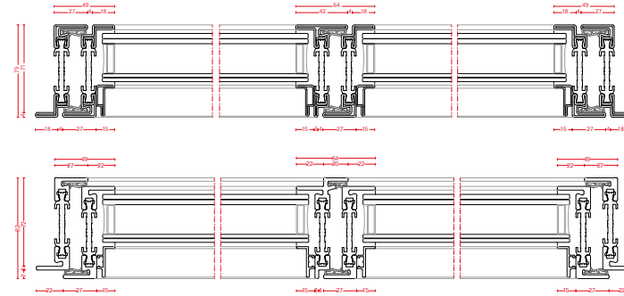
Finestra a due ante apertura interna
